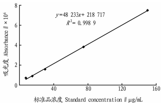
图 3 灵芝酸 A 标准品的标准曲线
